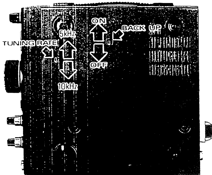
Ubicación de los Interruptores en la Tapa Inferior
