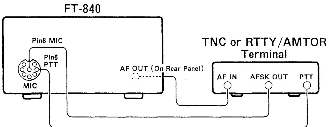
Interconexiones de Unidad Terminal RTTY/AMTOR & Paquete TNC
