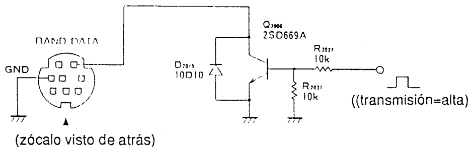
Conmutación T/R de Amp Lineal en el FT-840
