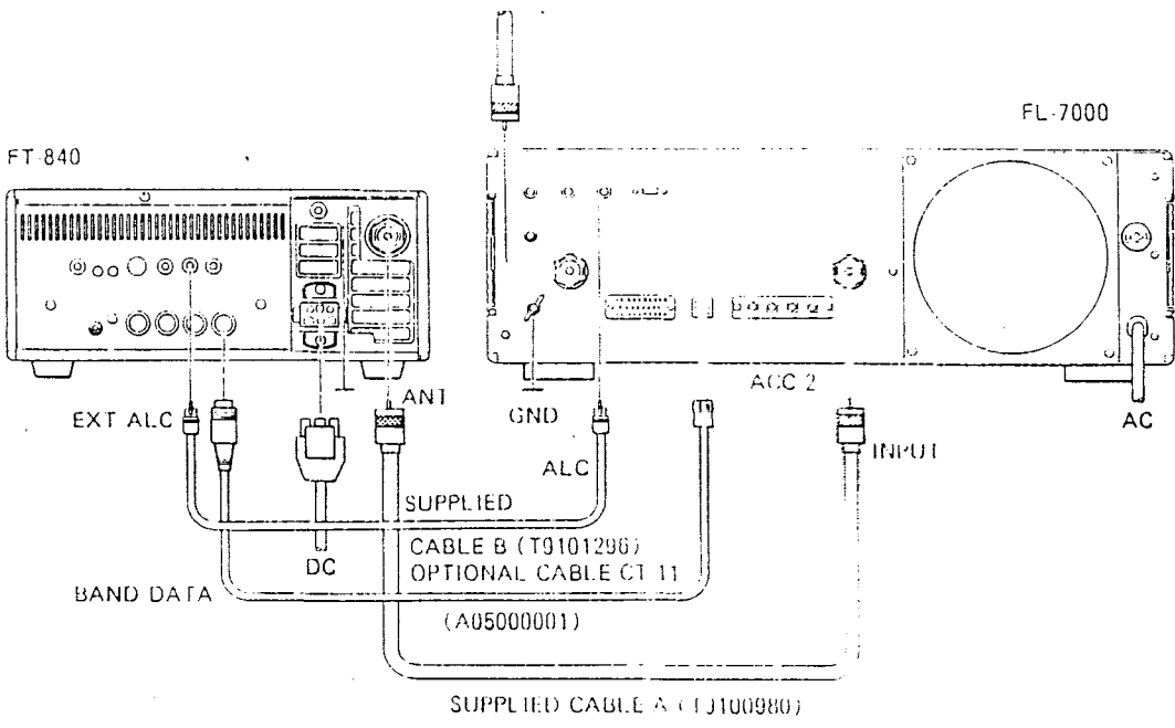
Amplificador Lineal FL-7000
