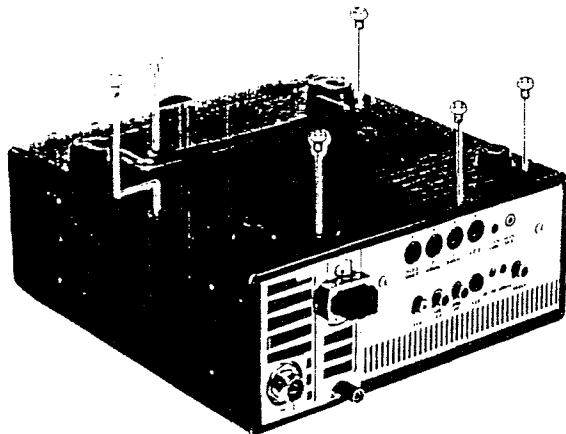
Ilus. 3: Como Quitar la Tapa Inferior
